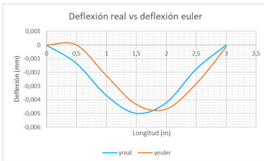
Fig 2. Deflexión real contra deflexión de Euler.
