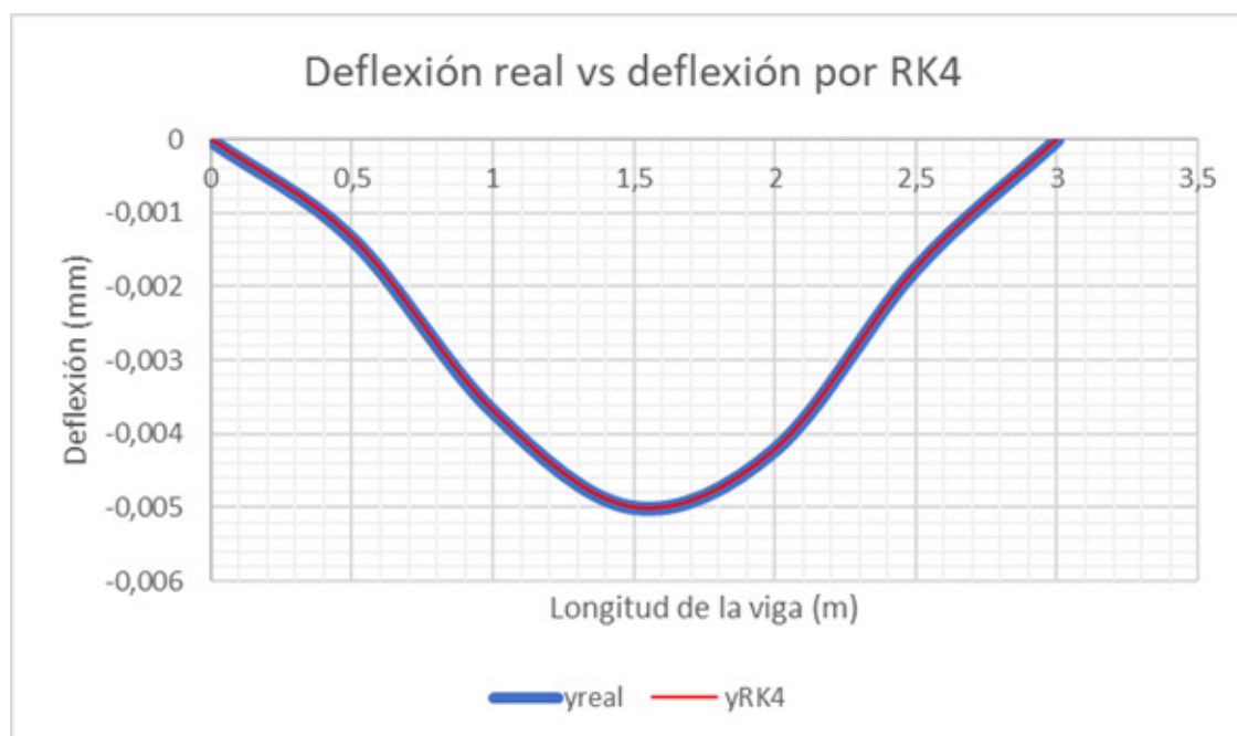
Fig 3. Deflexión real contra deflexión por Runge-Kutta.
