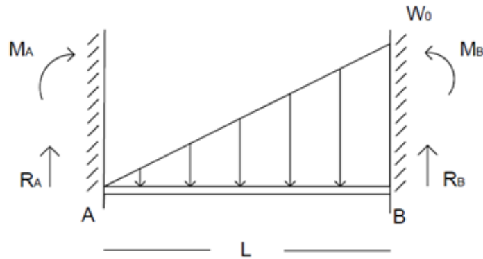
Fig 1. Viga estáticamente indeterminada con carga triangular creciente.
